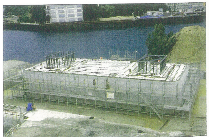
●Qマツト使用例(橋脚基礎フーチング)
