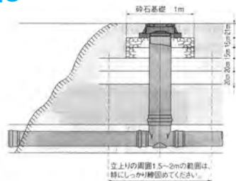
＜図3 鋳鉄製防護ふたの施工例＞
