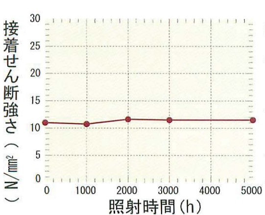
■照射時間と接着せん断強さ
