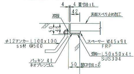
単板蓋 (受枠50mmの場合)
