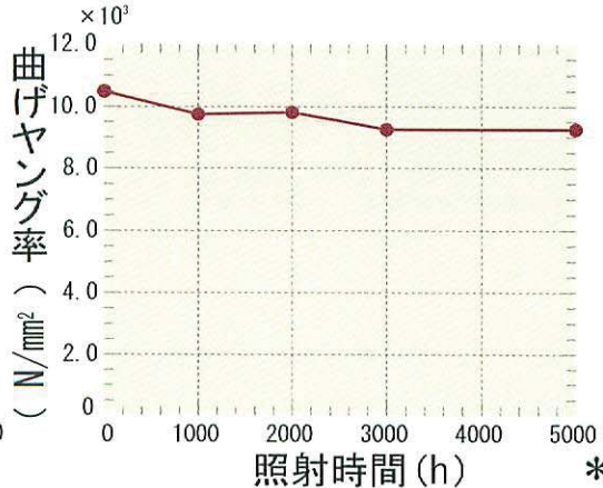
■照射時間と測定値の曲げヤング率
