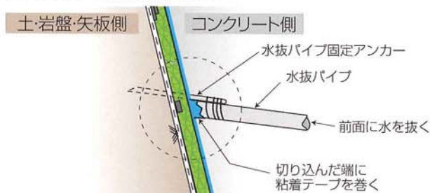
〈断面図〉 [パイプ差込部詳細図]
