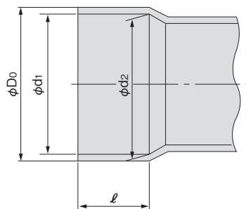
接着受口&lt;本管・取付け管用&gt;
