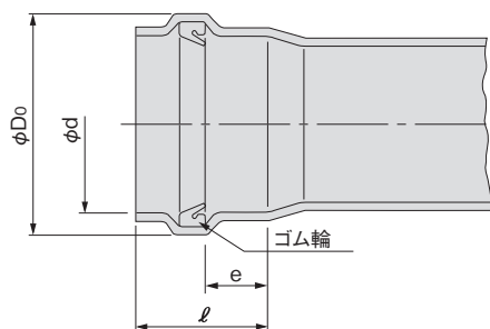
取付け管ゴム輪受口&lt;支管・取付け管用&gt;
