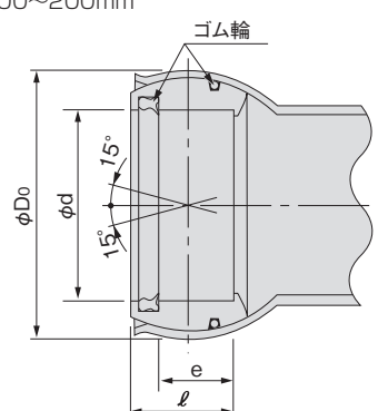
自在受口(取付け管ゴム輪受口)&lt;支管・取付け管用&gt;
