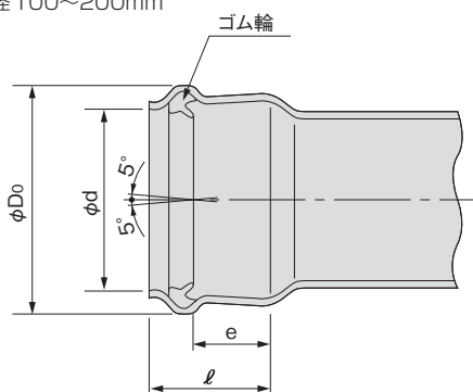
取付け管ゴム輪受口&lt;支管・取付け管用&gt;
