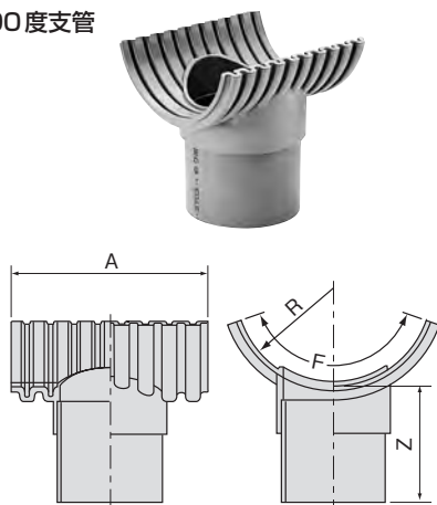
副管用90度支管
